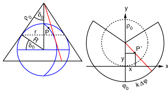
Slika 31.13 Stožčna konformna projekcija. Projekcija je primerna za prikaz dežel v zmernem pasu.
