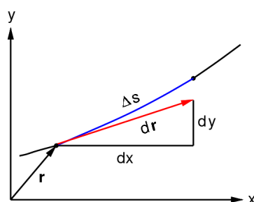
Slika 31.5 Ločni element krivulje. Njegova dolžina je limitno enaka spremembi vektorja lege.
